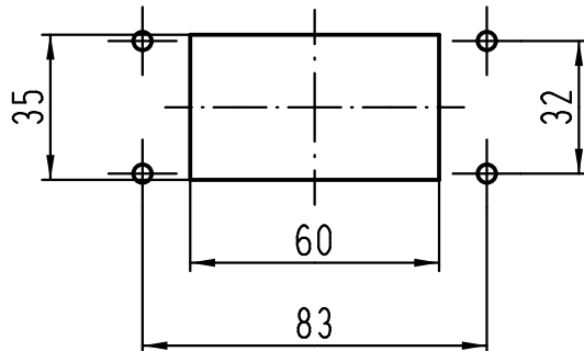
1:2 Montageausschnitt panel cut out
