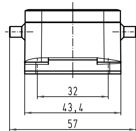
1:2 Montageausschnitt panel cut out
