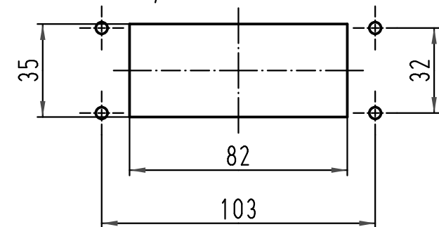
1:2 Montageausschnitt panel cut out
