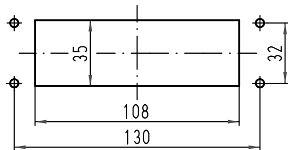
Montageausschnitt panel cut out 1:2
