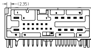
30700-5241/30700-5245 POLARIZATION 'B'
