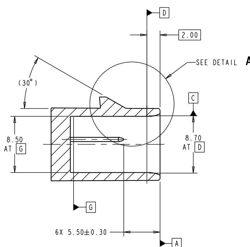
SECTION D-D
