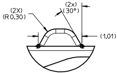
DETAIL 1 SCALE 25:1
