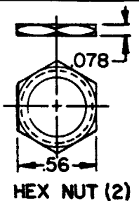
HEX NUT (2)
