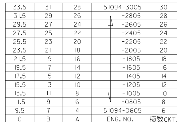
ハウジング アッセンブリ装着状態図 FIGURE OF HOUSING ASSEMBLY WHEN ASSEMBLED
