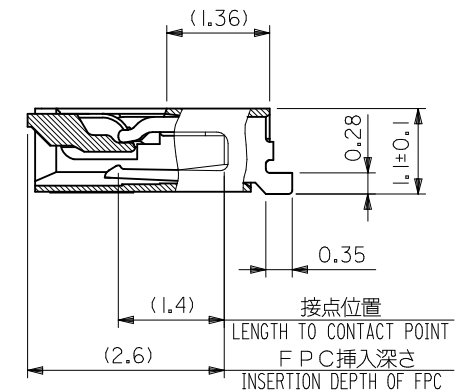
断面 W-W SECT. W-W 偶数極 (EVEN CKT)
