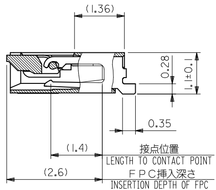
断面 V-V SECT. V-V 奇数極 (ODD CKT)
