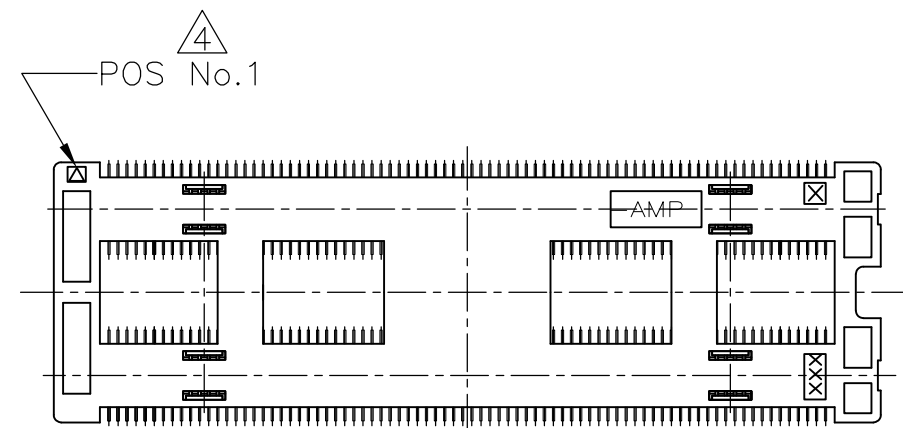
D-D (SCALE 2:1)
