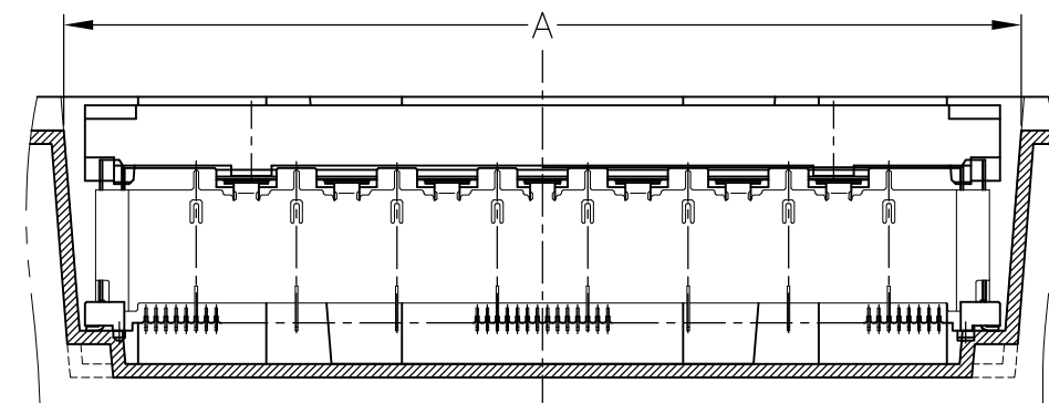
D-D (SCALE 2:1)
