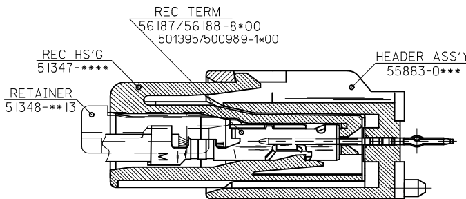
嵌合断面図
