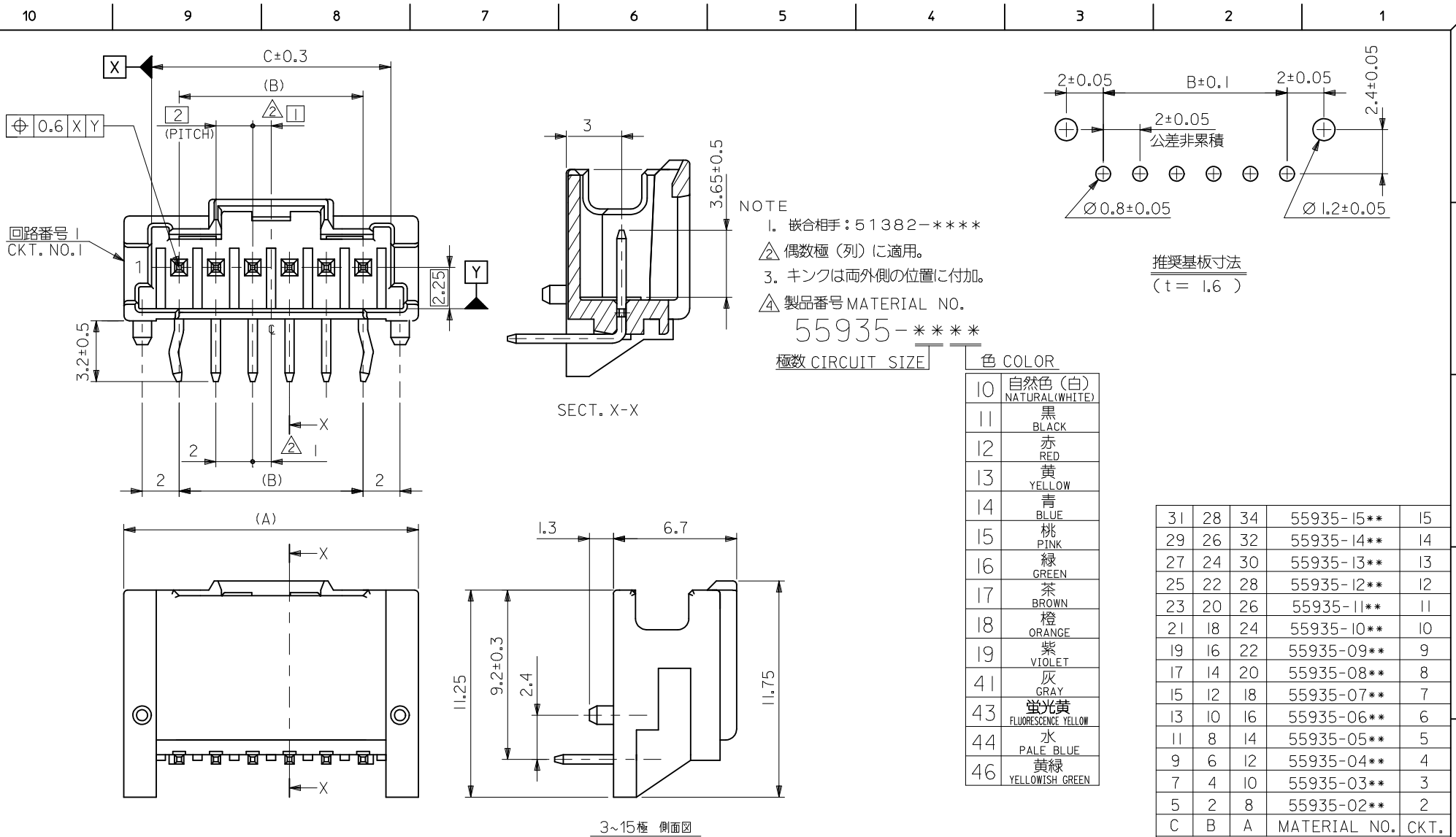
3~15極 側面図
