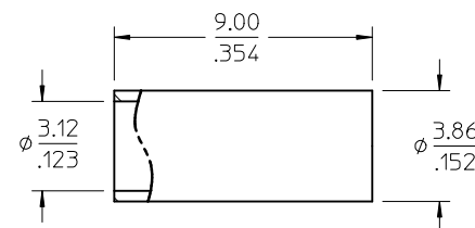
FERRULE
