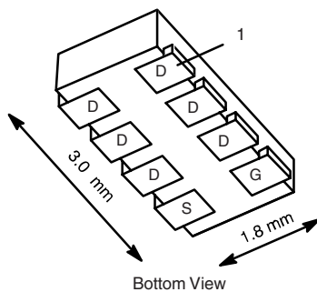
1206-8 ChipFET®
