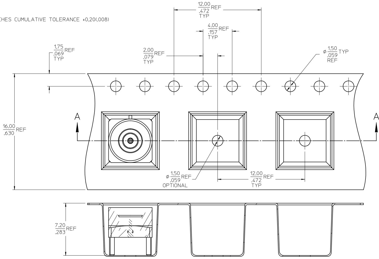
SECTION A-A
