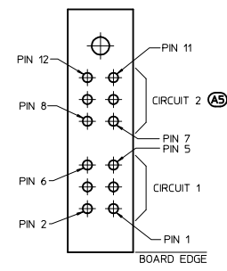
PINOUT DETAIL SCALE: 4:1
