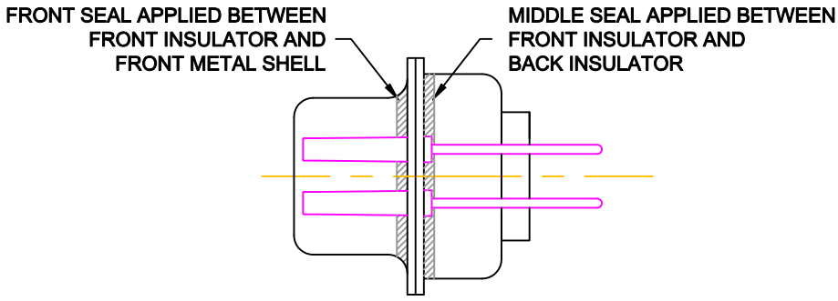
DETAIL A-A
