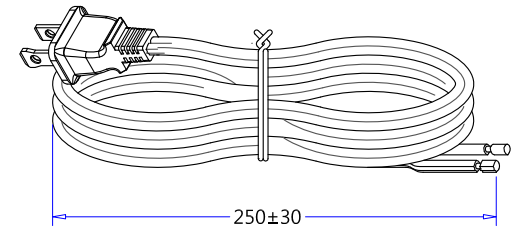
B-C3 扎線圖示 (Tied Loop Hank Detail)
