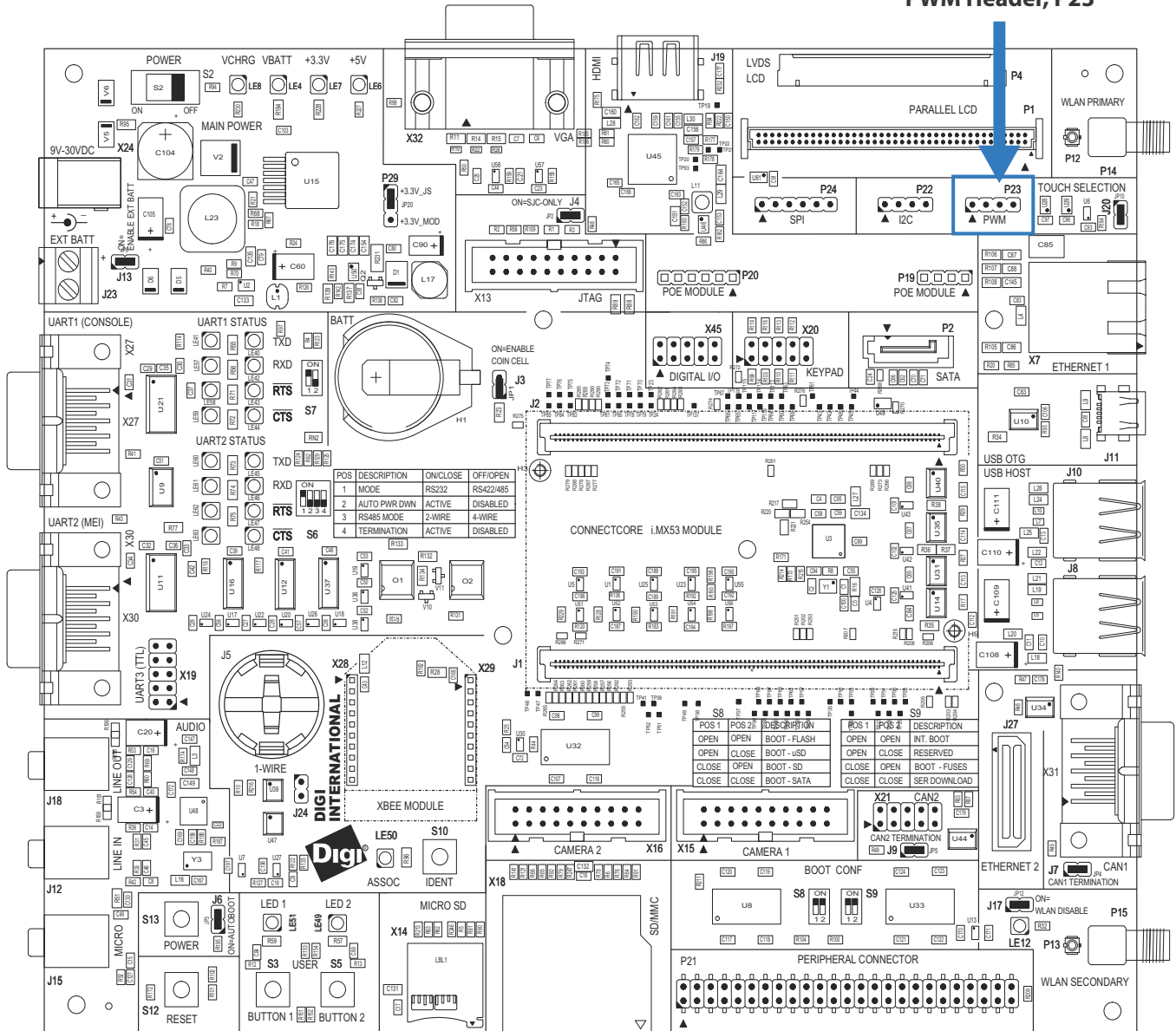
PWM Header, P23
