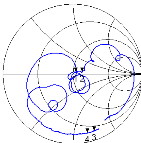
Fig.5 Input Impedance
