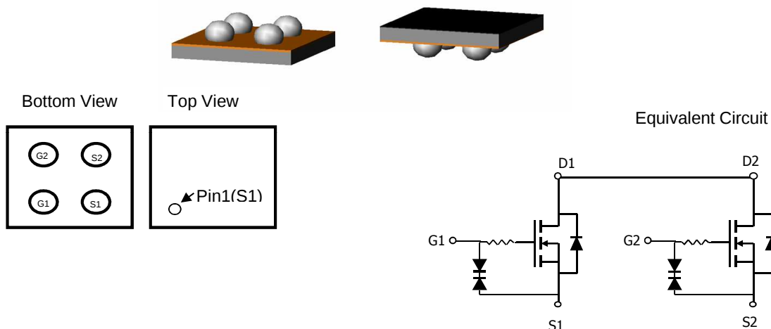
WLCSP 1.57x1.57_4
