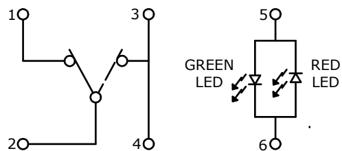
SCHEMATIC ▲ SPDT
