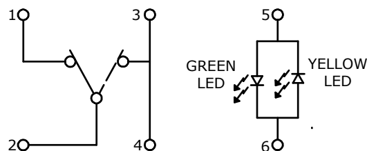
SCHEMATIC SPDT
