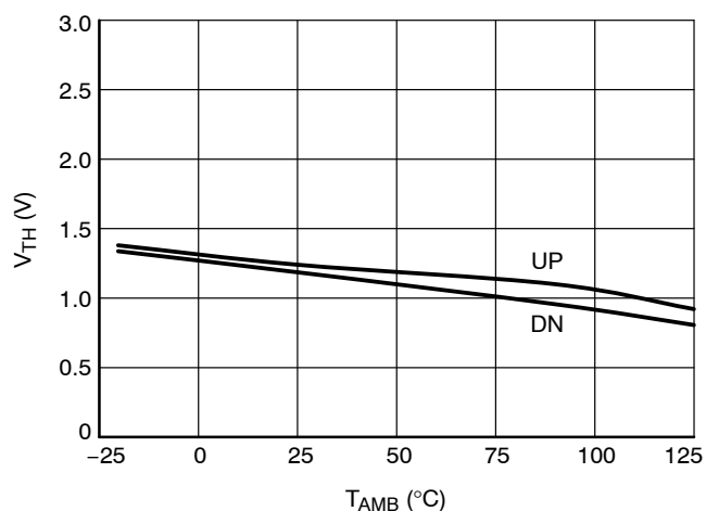
Figure 15. TS POR Threshold Voltage (Rev. C)
