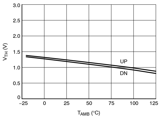
Figure 17. SPD POR Threshold Voltage (Rev. C)
