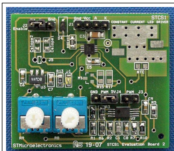
STEVAL-ILL014V1
