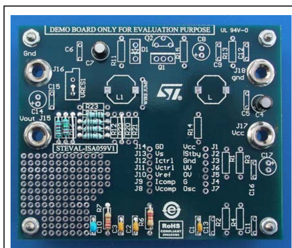
STEVAL-ISA059V1
