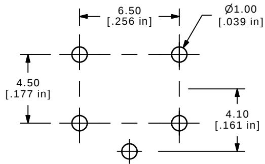
P.C. LAYOUT
