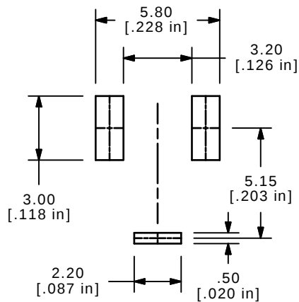
P.C.B. LAYOUT
