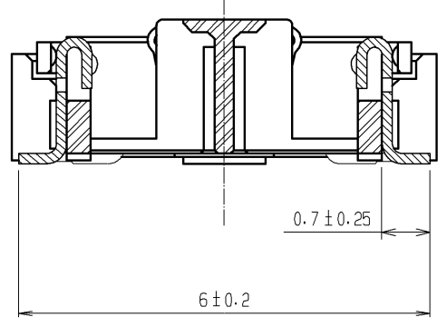
B-B (10 : 1)
