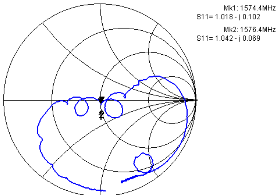
Fig.5 Input impedance
