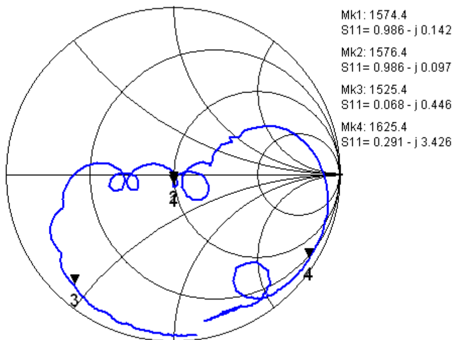
Fig.5 Input impedance
