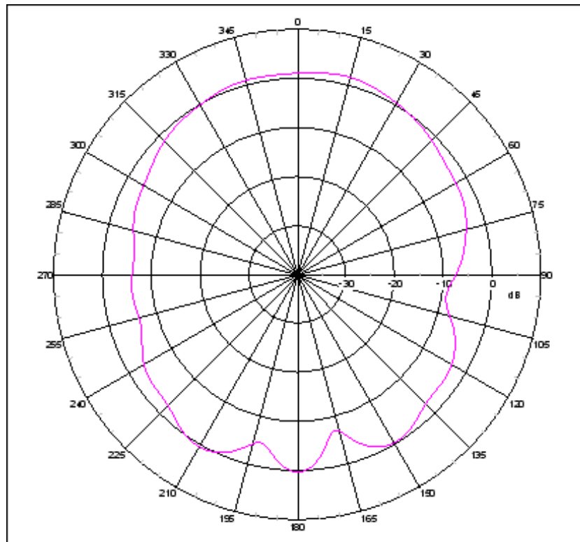
YZ-plane Free Space @1602MHz
