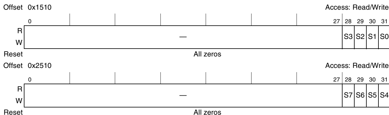
Figure 9-30. Message Status Register (MSR)
