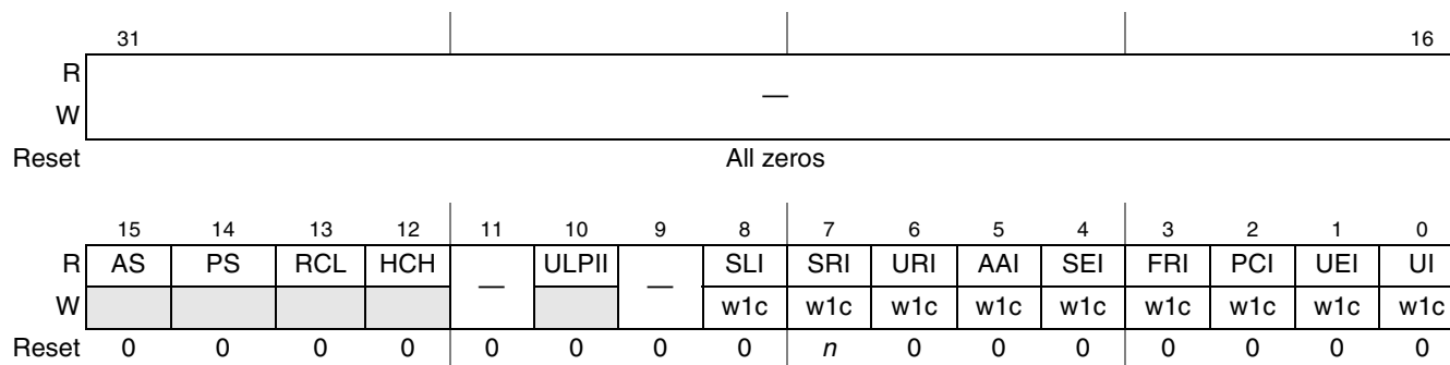
Figure 21-9. USB Status Register (USBSTS)
