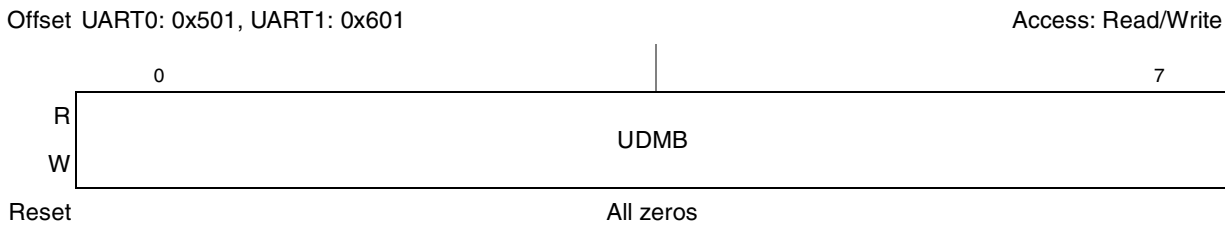
Figure 12-4. Divisor Most Significant Byte Registers (UDMB0, UDMB1)
