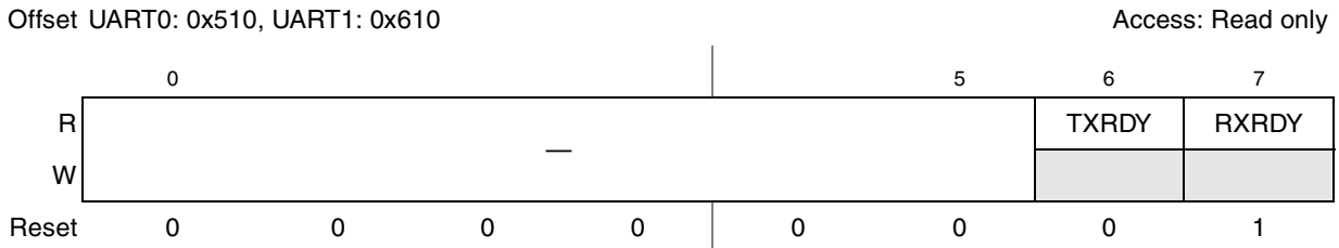
Figure 12-15. DMA Status Register (UDSR)
