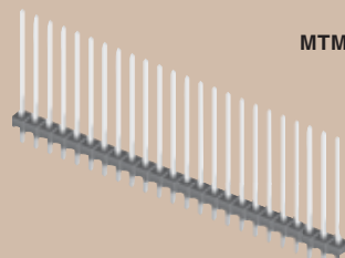
MTMM-124-14-L-S-600
