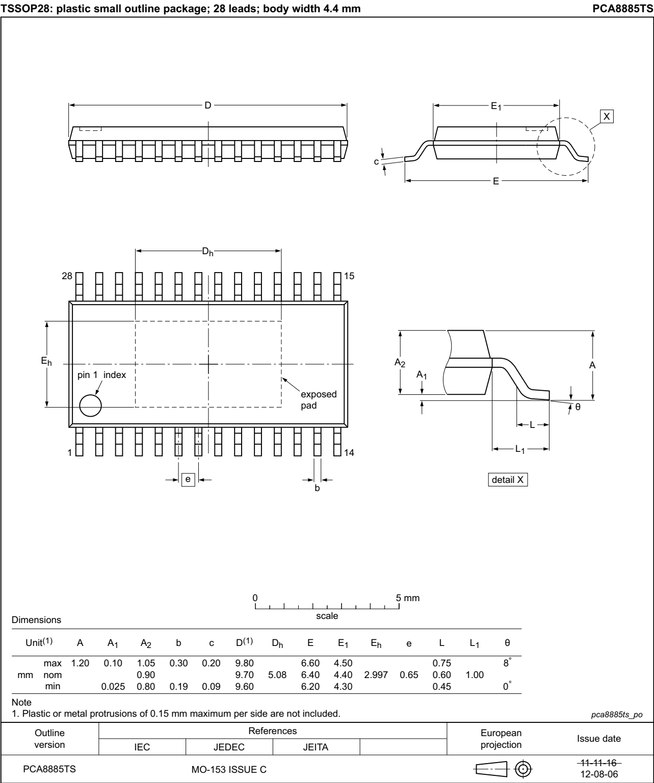
Fig 26. Package outline PCA8885TS (TSSOP28)
