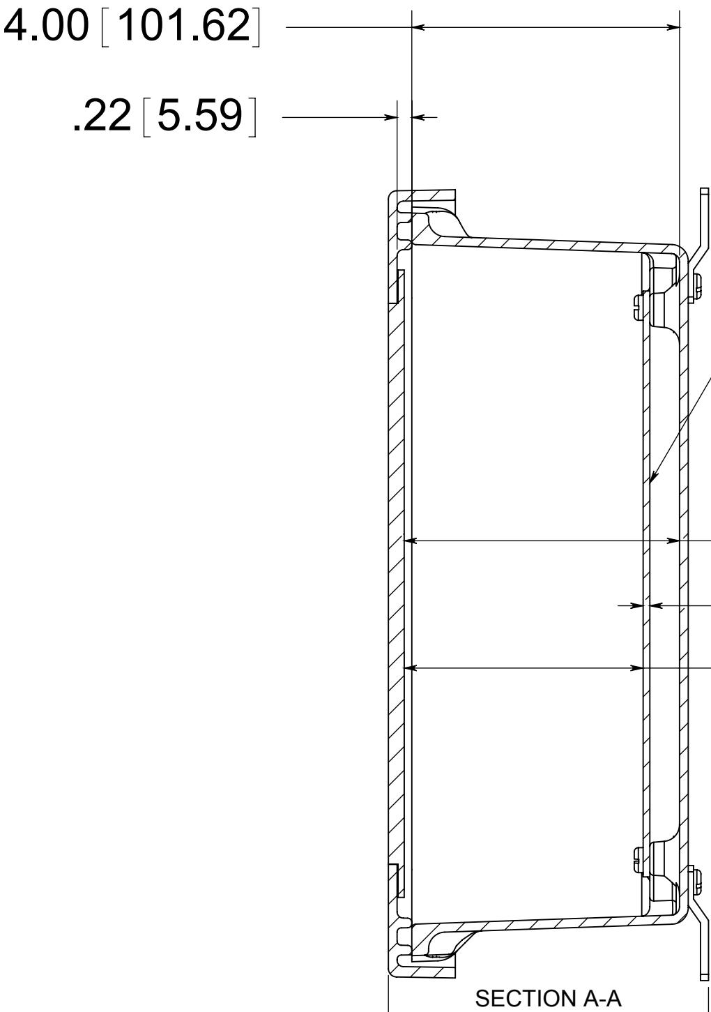
SECTION A-A
