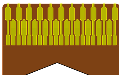
水平挿入 Straight Insertion
