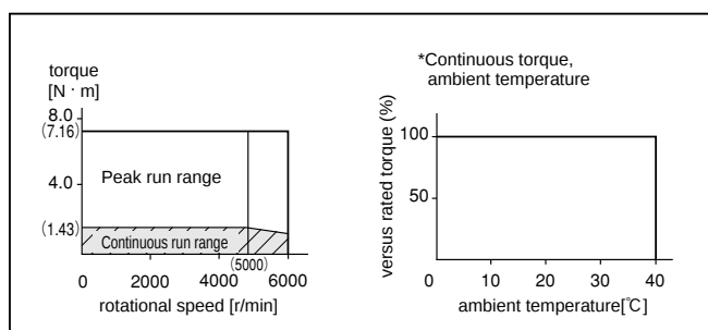
MAMA082□1□
