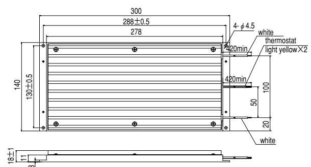
DV0P4285
