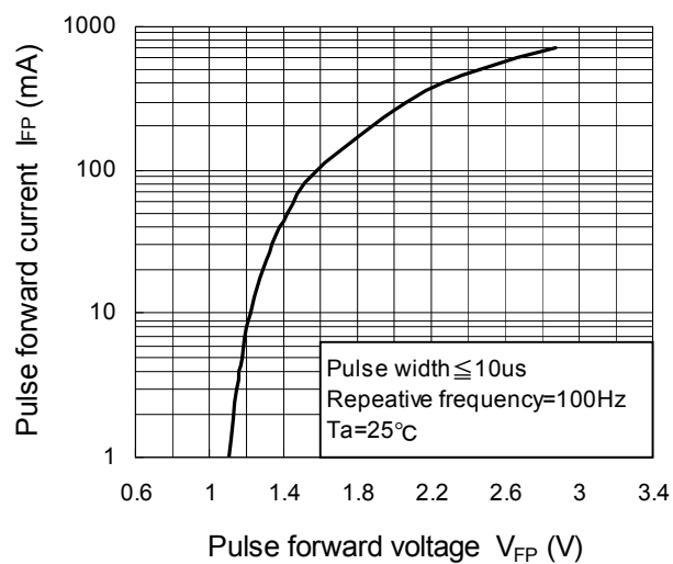
I_{FP} - V_{FP}
