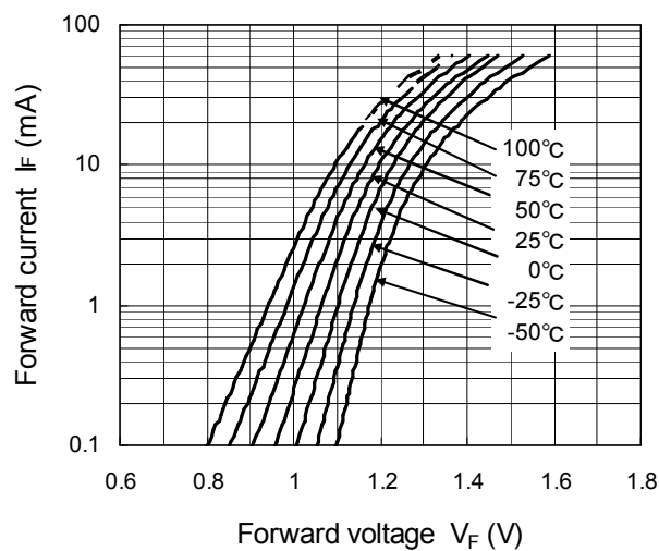
I_{FP} - V_{FP}
