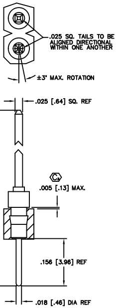
FIG. 11 TERMINAL STYLE -D-1-1 T-1S4-1-1-X
