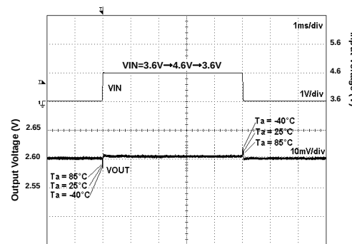
Fig 154. VIN Response
