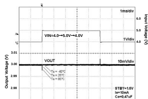
Fig 232. VIN Response
