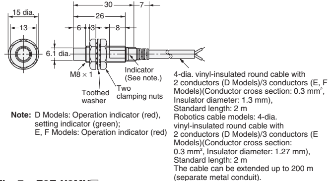
Fig. 7: E2E-X2MY□
