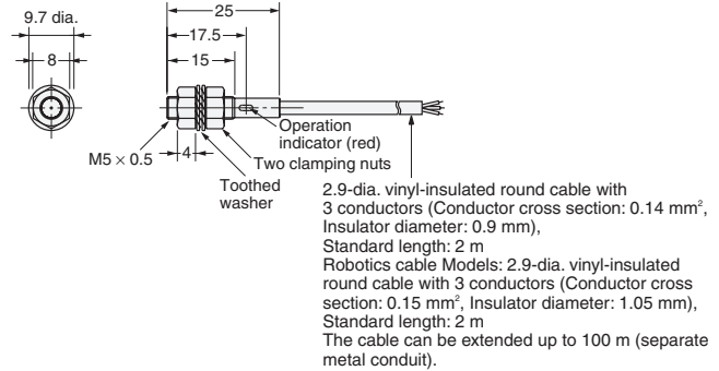
Fig. 3: E2E-X1□□
