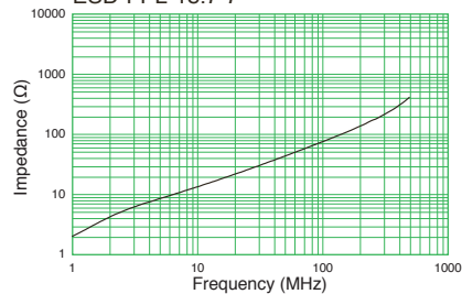
ESD-FPL-18.7-7
