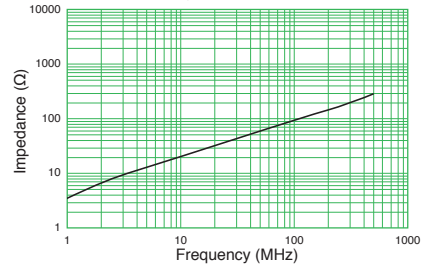
ESD-FPD-50,50-1
