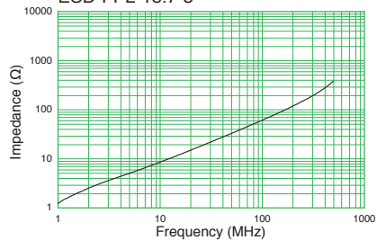
ESD-FPL-18.7-3
