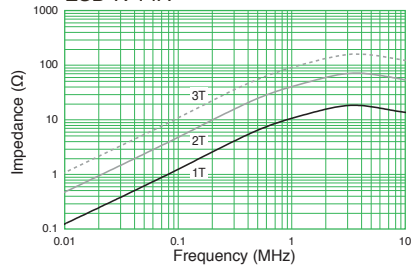
ESD-R-19S/19/19B
