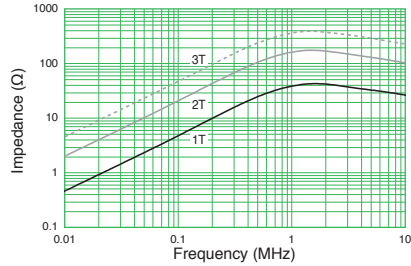
ESD-R-31-P
