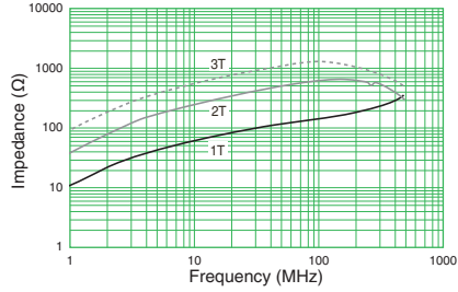
ESD-R-12E
