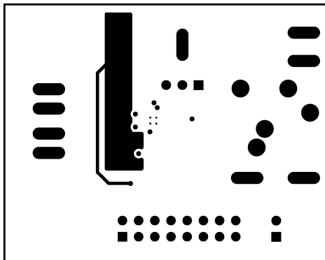
Figure 32. Layer 3 (V DD )
