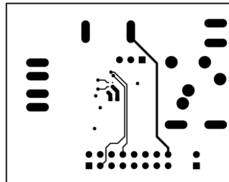
Figure 33. Bottom Layer
