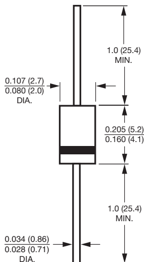
DO-204AL (DO-41)
