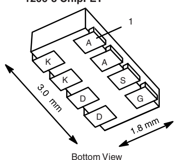
1206-8 ChipFET®
