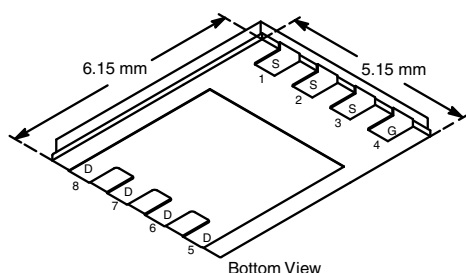
PowerPAK® SO-8
