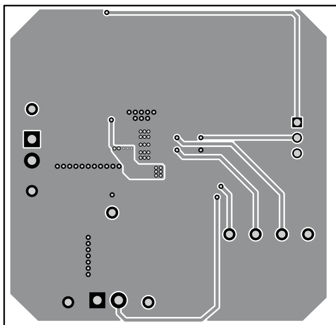
Figure 18. Bottom Layer
