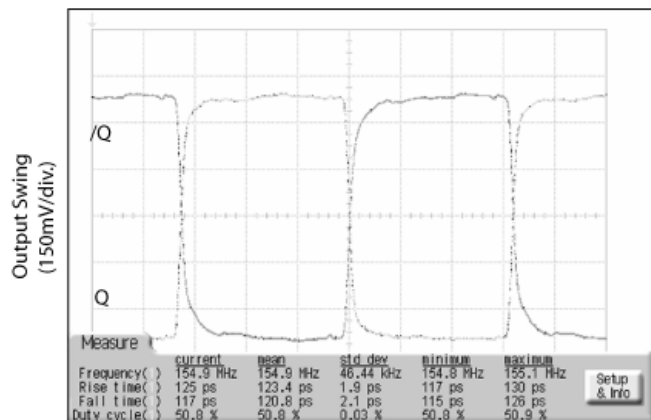
155MHz Output
