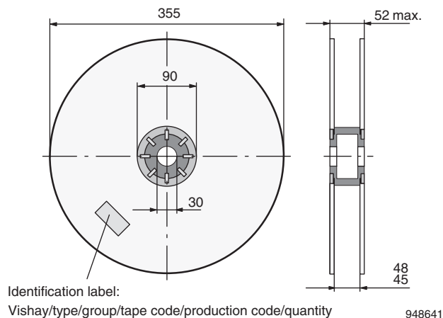
Fig. 24 - Reel Dimensions
